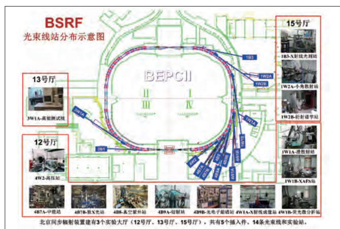
⊙ BSRF 光束线站分布示意图
