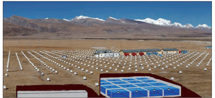
① 西藏 AS \gamma 实验复合式阵列（表面阵列 + 地下水切伦科夫阵列）
