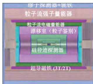
④ 新概念的 CEPC 第四探测器概念设计图
