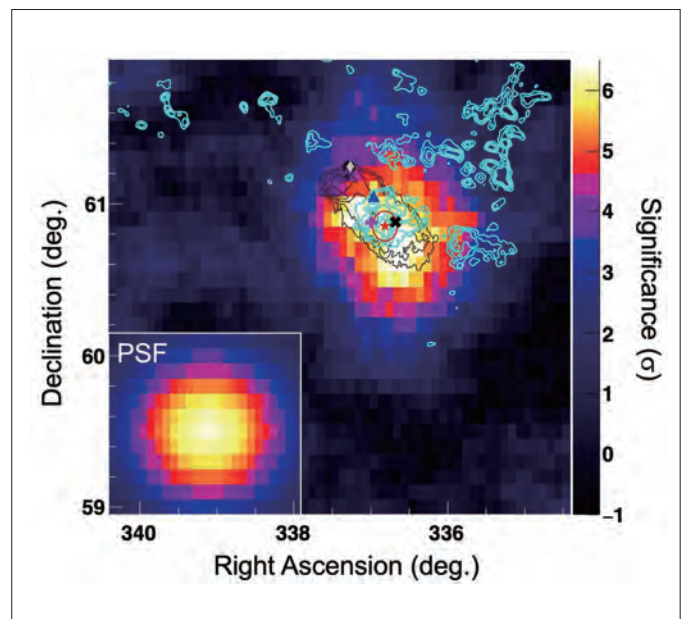
① 西藏 AS \gamma 实验观测到超新星遗迹（SNR）G106.3+2.7 附近 10 TeV 以上的伽马辐射图像，伽马辐射能量延续到 100 TeV 以上，该结果发表在《Nature Astronomy》（自然天文）
