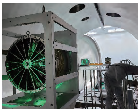
① EP 卫星 FXT 聚焦镜组件
