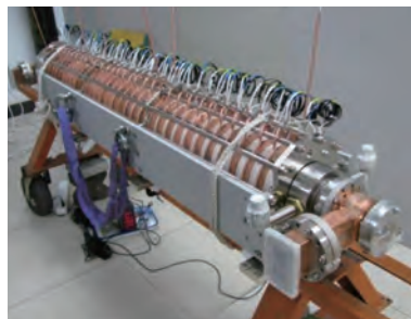
④ 9MeV 加速器射线源工业 CT (上左)、工业辐照用 10MeV 电子加速器 (上中)、医用加速器加速管 (上右)
