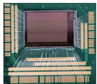
④ 高空间分辨 (3-5 微米位置分辨率) 的硅像素探测器芯片
