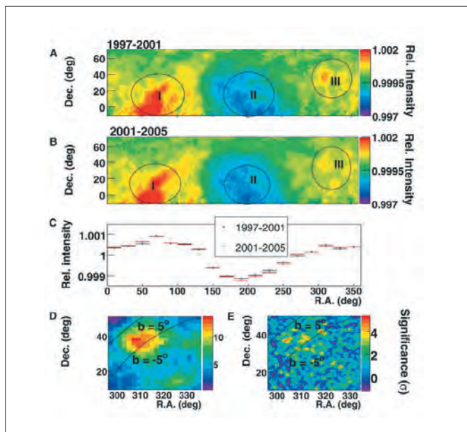
① 依据“西藏 AS \gamma ”所获得的近四百亿观测事例，中日物理学家合作发表的结果
